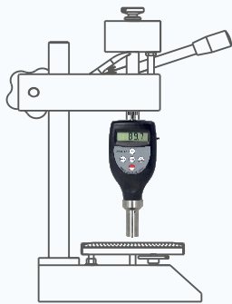
邵氏硬度计测试支架
